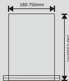
Sewn bag
